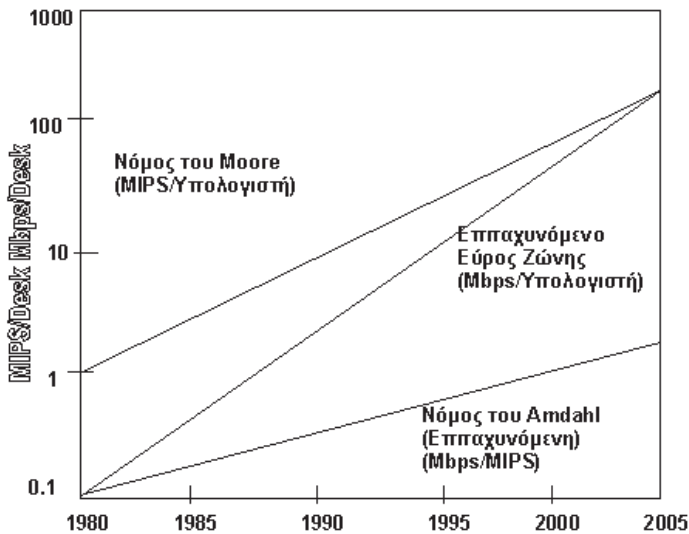
Σχήμα 1.4: Καμπύλες Moore και αύξησης επικοινωνιακού εύρους ζώνης
